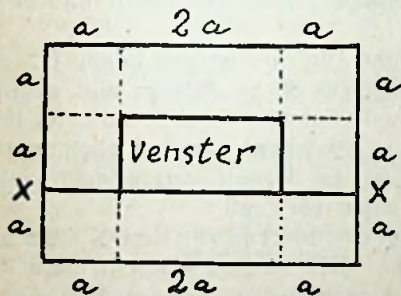
Fig. 3. Afmetingen en verhoudingen van de Kern; bij X is de luchtspleet.
